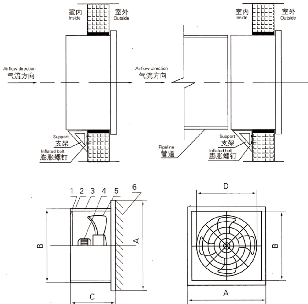
YTBZ系列壁式风机外型尺寸及安装孔尺寸表
